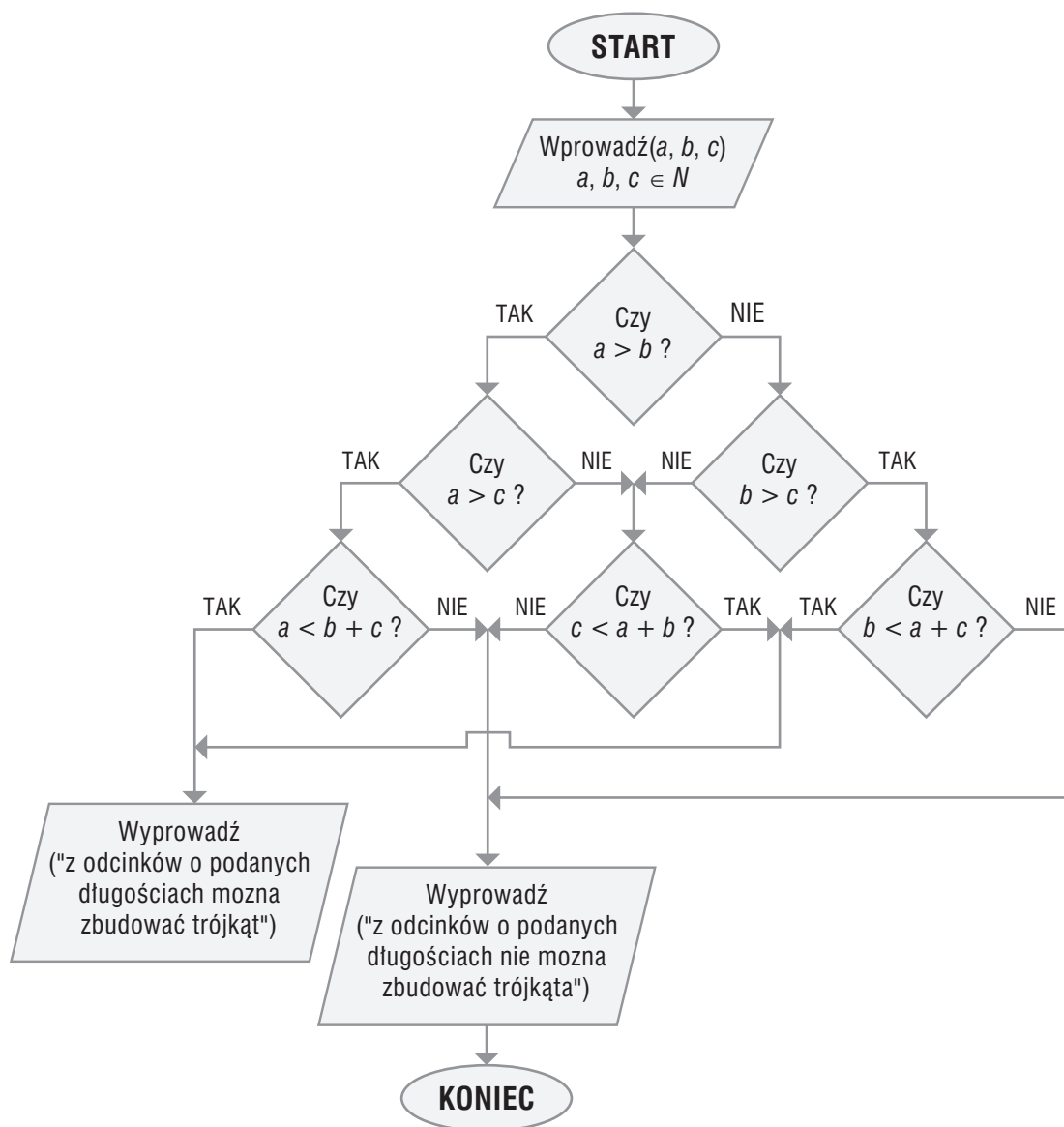
Schemat blokowy algorytmu sprawdzania warunku trójkąta
